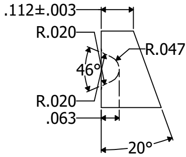
GASKET GROOVE 14WMP-2 1/2"
